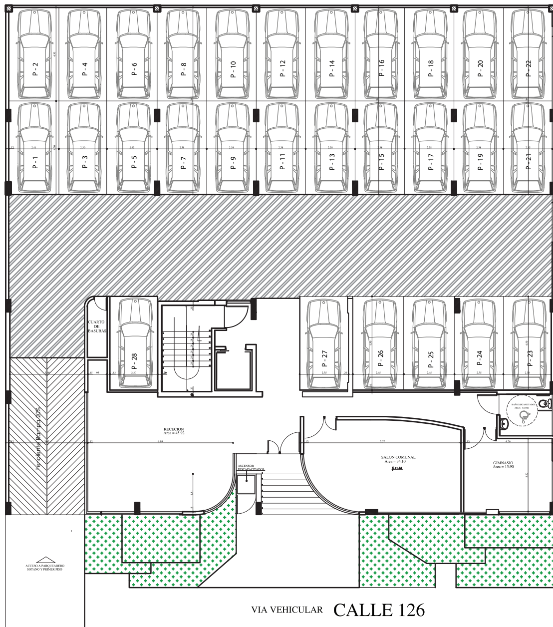
PLANTA PRIMER PISO ESC: 1:50
